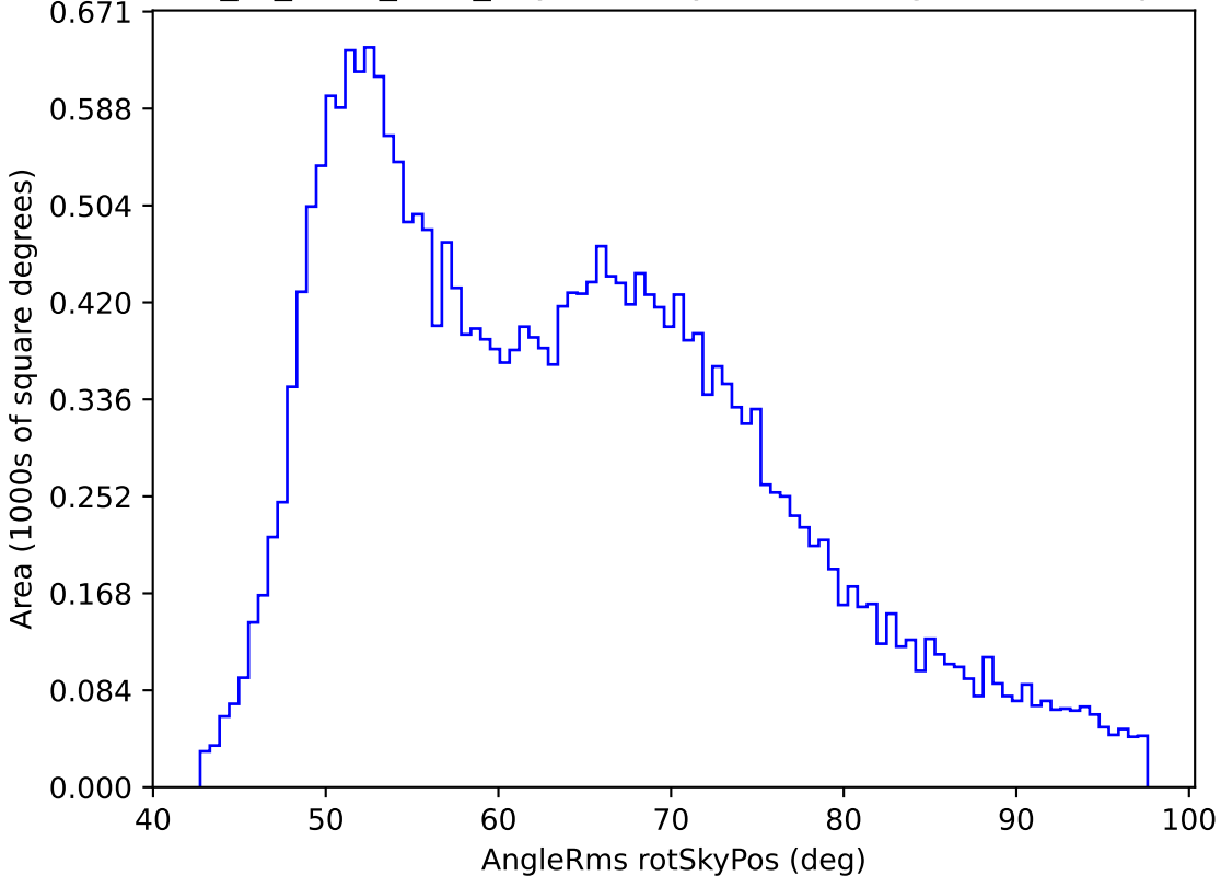
extra_ss_neo7_v3.4_10yrs All sky r band: AngleRms rotSkyPos
