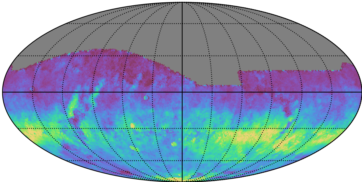
extra_ss_neo7_v3.4_10yrs All sky i band: AngleRms rotSkyPos
