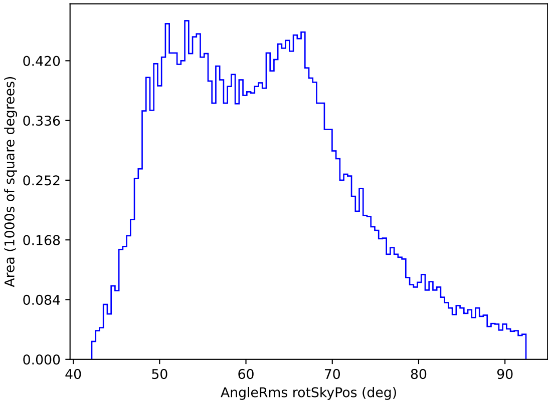
extra_ss_neo7_v3.4_10yrs All sky i band: AngleRms rotSkyPos
