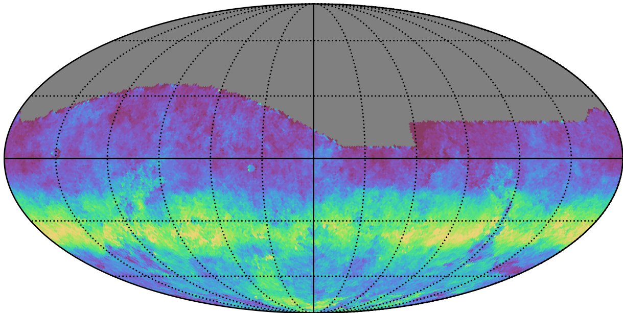
extra_ss_neo7_v3.4_10yrs All sky g band: AngleRms rotSkyPos
