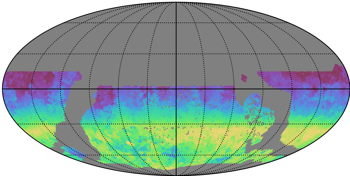
extra_ss_neo7_v3.4_10yrs WFD z band: AngleRange rotSkyPos
