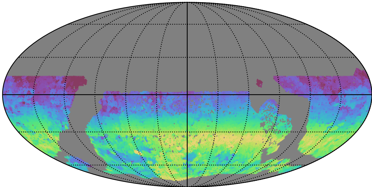
extra_ss_neo7_v3.4_10yrs WFD y band: AngleRange rotSkyPos
