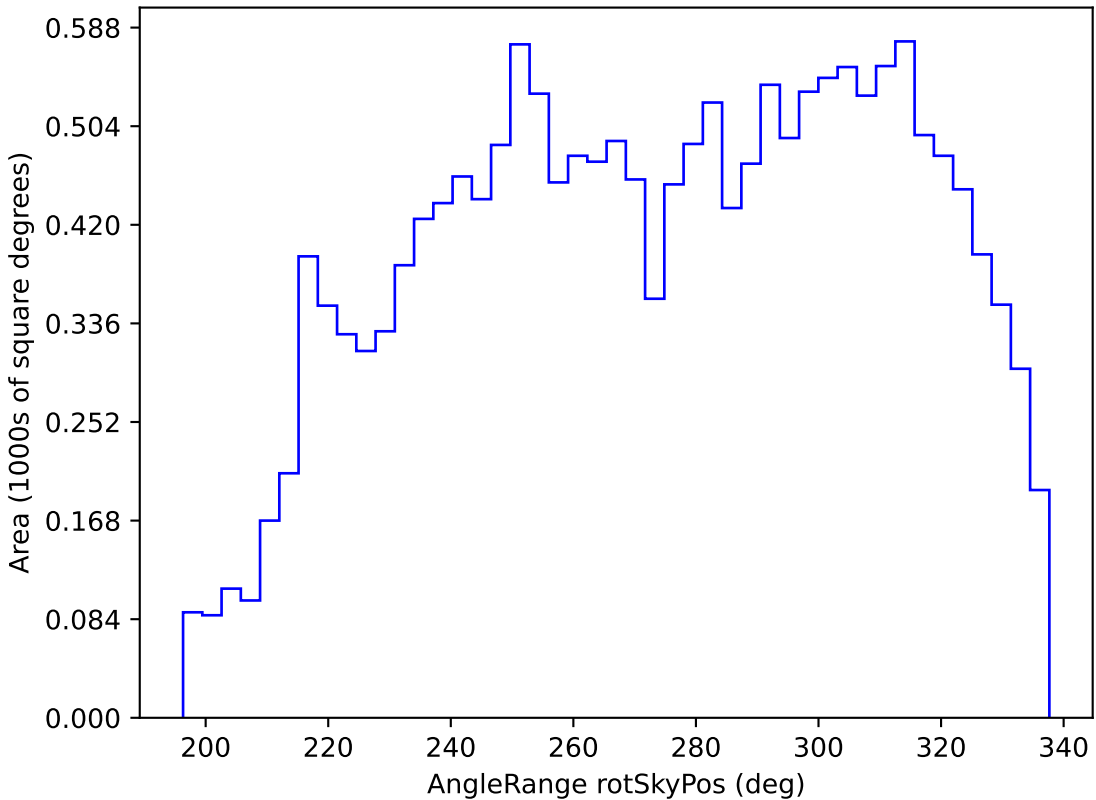
extra_ss_neo7_v3.4_10yrs WFD y band: AngleRange rotSkyPos
