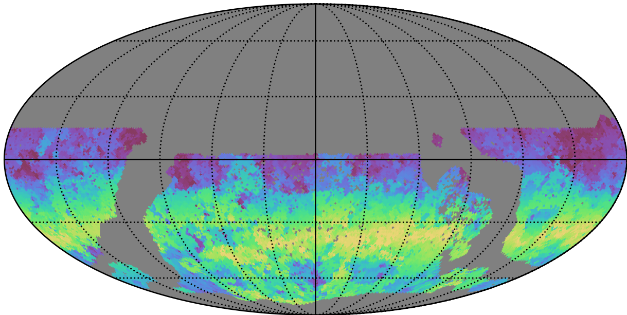
extra_ss_neo7_v3.4_10yrs WFD u band: AngleRange rotSkyPos
