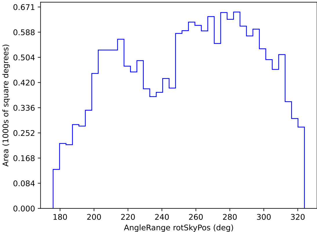
extra_ss_neo7_v3.4_10yrs WFD u band: AngleRange rotSkyPos
