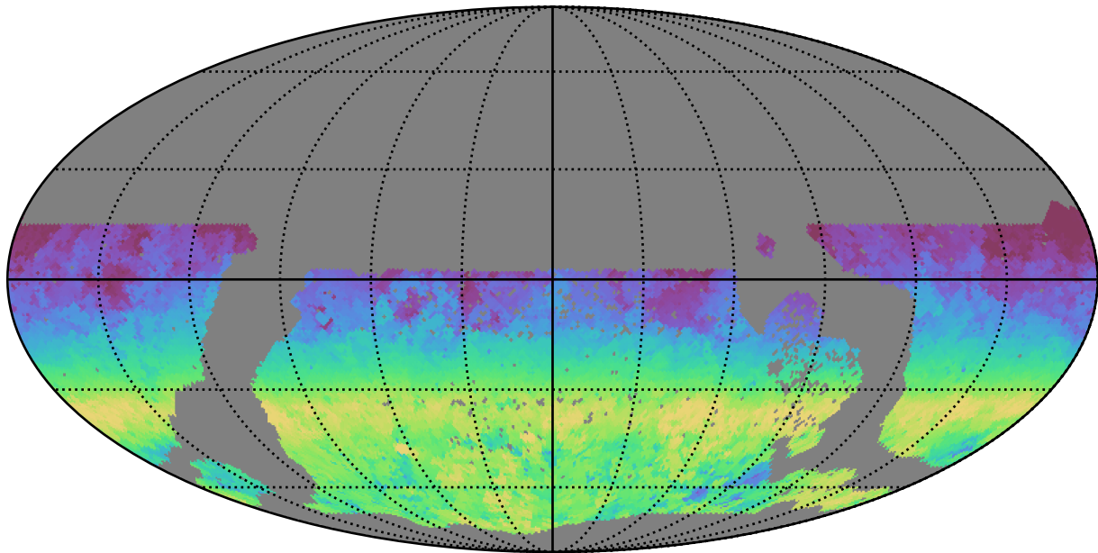
extra_ss_neo7_v3.4_10yrs WFD r band: AngleRange rotSkyPos
