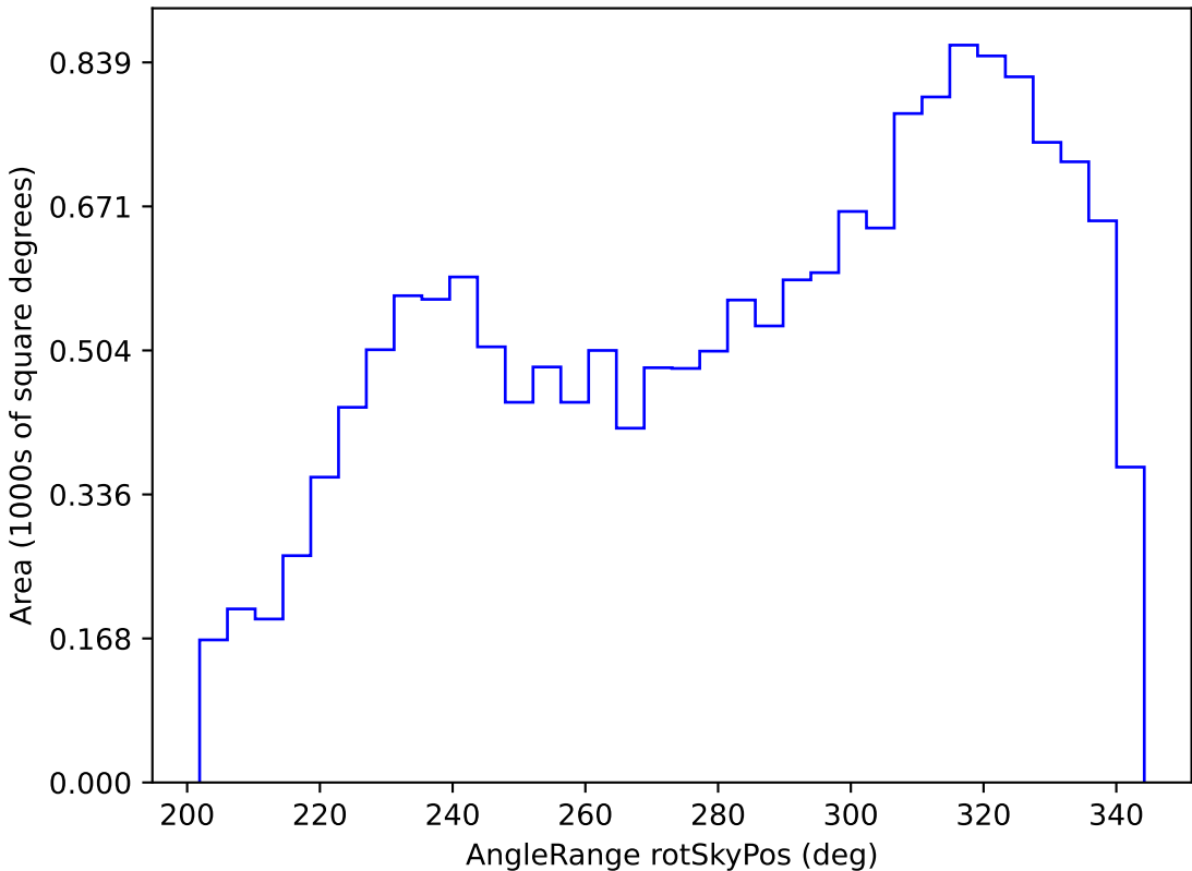
extra_ss_neo7_v3.4_10yrs WFD r band: AngleRange rotSkyPos
