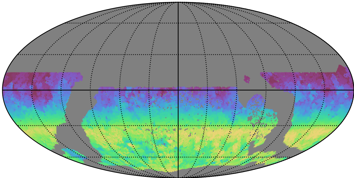
extra_ss_neo7_v3.4_10yrs WFD i band: AngleRange rotSkyPos
