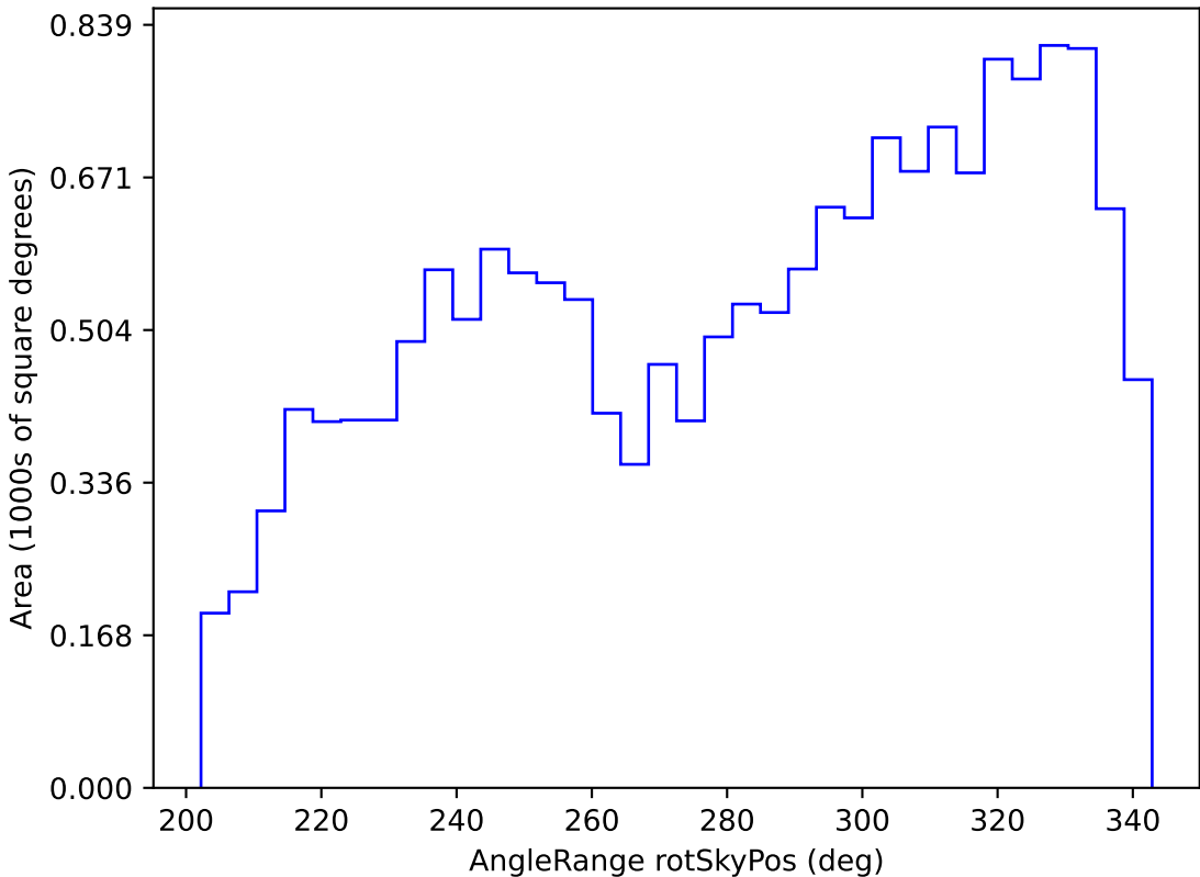
extra_ss_neo7_v3.4_10yrs WFD i band: AngleRange rotSkyPos
