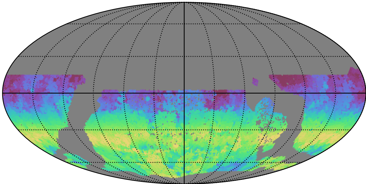
extra_ss_neo7_v3.4_10yrs WFD g band: AngleRange rotSkyPos
