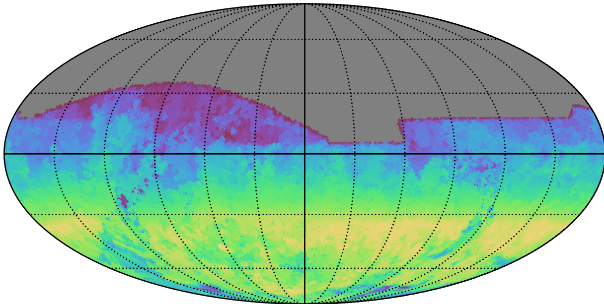
extra_ss_neo7_v3.4_10yrs All sky z band: AngleRange rotSkyPos
