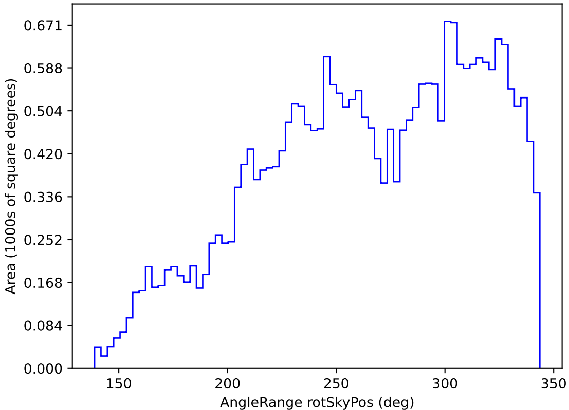
extra_ss_neo7_v3.4_10yrs All sky z band: AngleRange rotSkyPos
