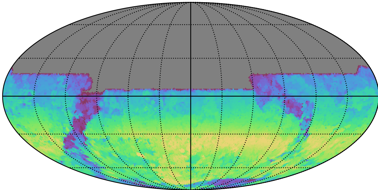
extra_ss_neo7_v3.4_10yrs All sky y band: AngleRange rotSkyPos
