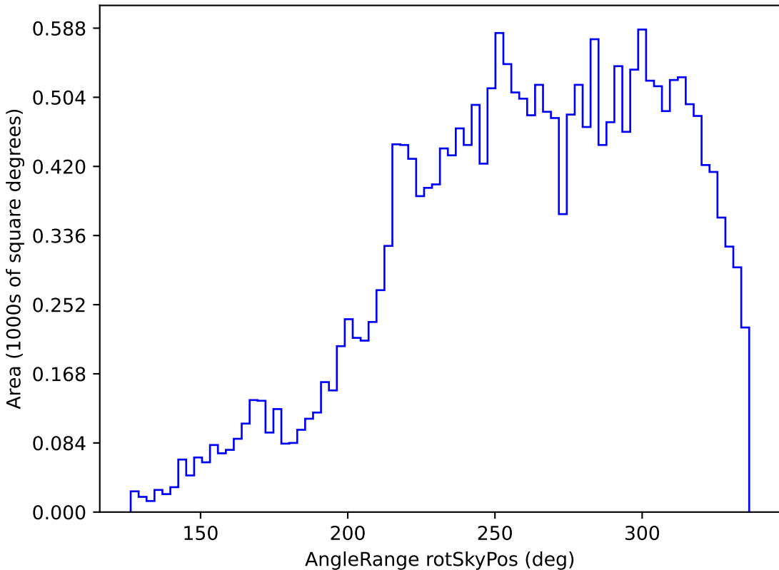
extra_ss_neo7_v3.4_10yrs All sky y band: AngleRange rotSkyPos
