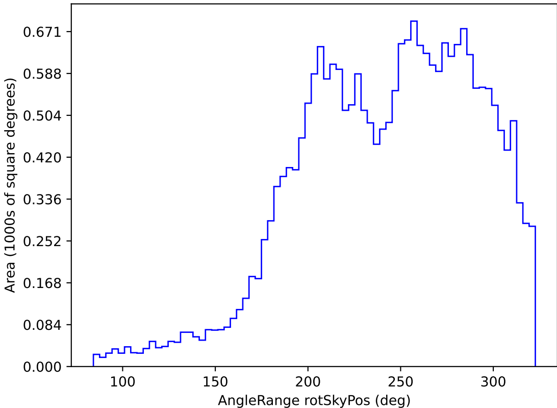
extra_ss_neo7_v3.4_10yrs All sky u band: AngleRange rotSkyPos
