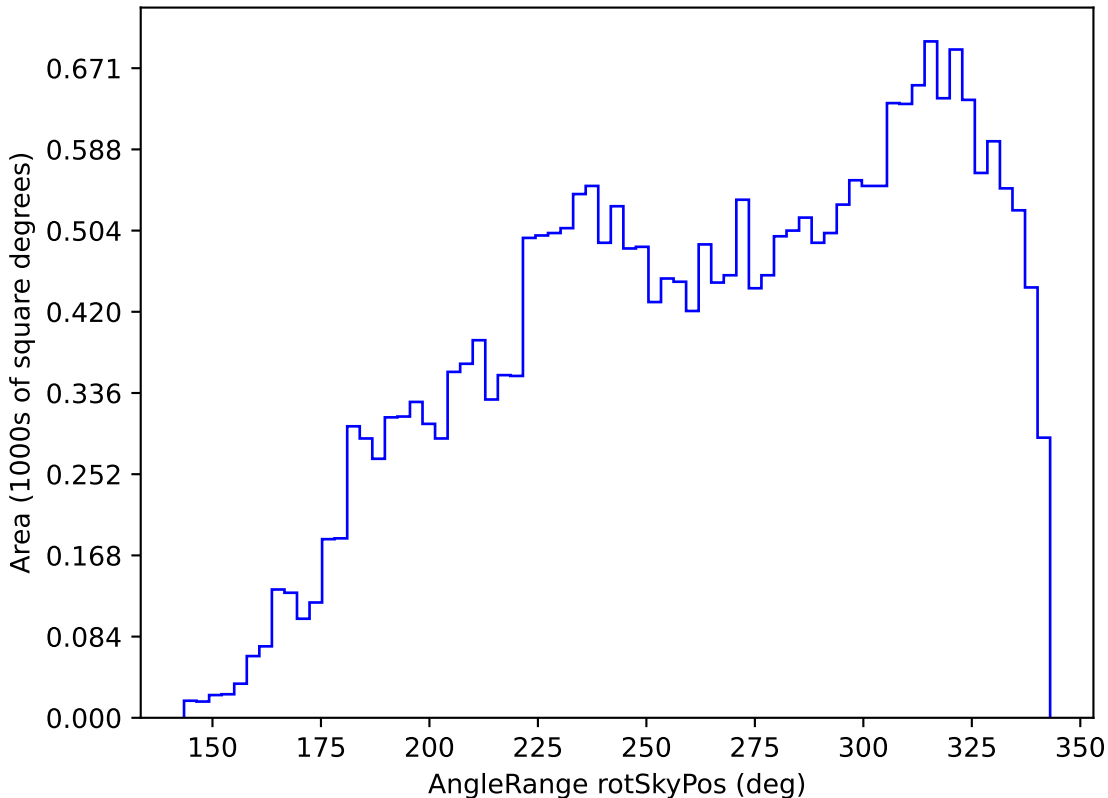
extra_ss_neo7_v3.4_10yrs All sky r band: AngleRange rotSkyPos
