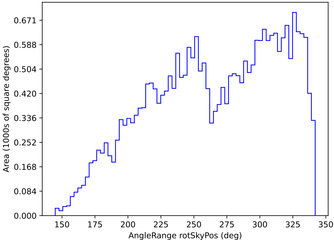
extra_ss_neo7_v3.4_10yrs All sky i band: AngleRange rotSkyPos
