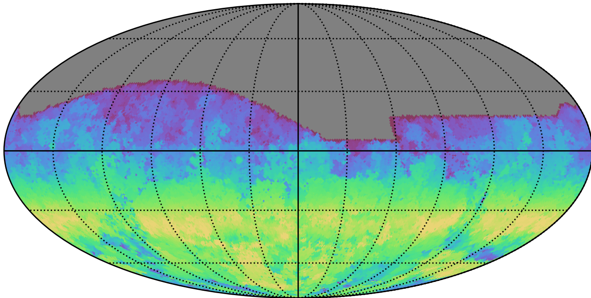
extra_ss_neo7_v3.4_10yrs All sky g band: AngleRange rotSkyPos
