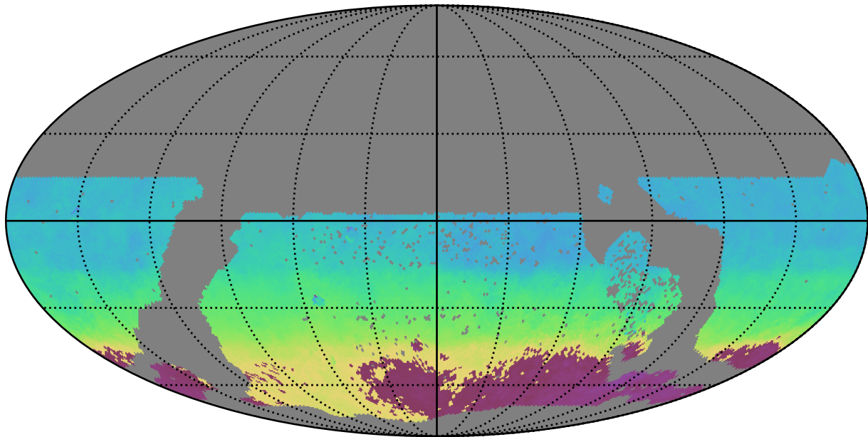
extra_ss_neo7_v3.4_10yrs WFD z band: AngleMean rotSkyPos
