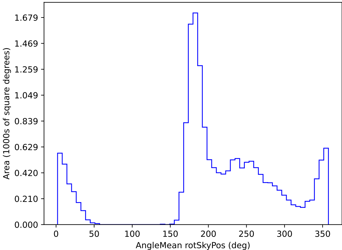
extra_ss_neo7_v3.4_10yrs WFD z band: AngleMean rotSkyPos
