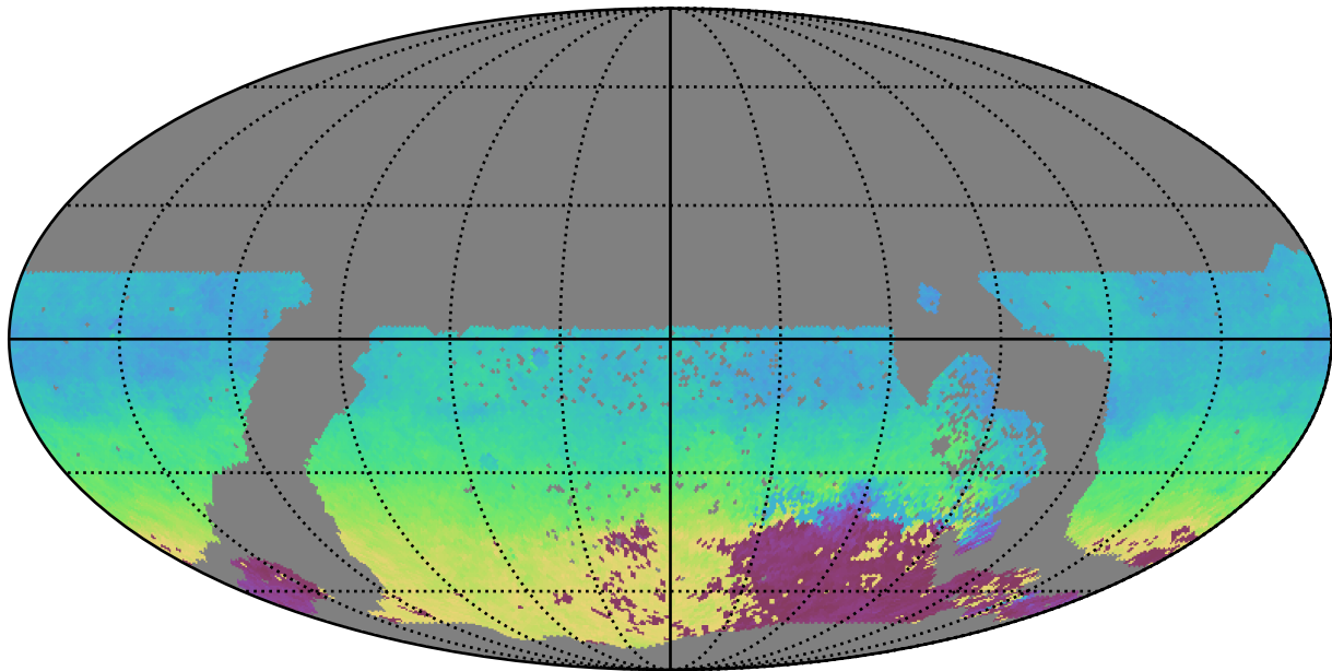
extra_ss_neo7_v3.4_10yrs WFD u band: AngleMean rotSkyPos
