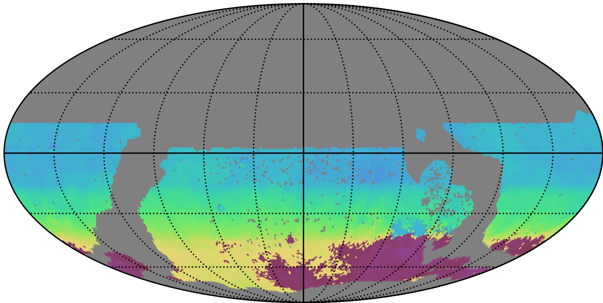
extra_ss_neo7_v3.4_10yrs WFD r band: AngleMean rotSkyPos
