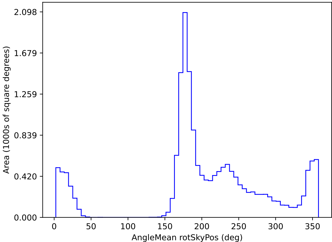
extra_ss_neo7_v3.4_10yrs WFD r band: AngleMean rotSkyPos
