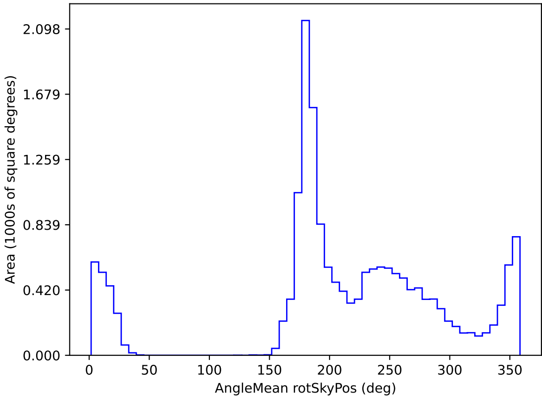
extra_ss_neo7_v3.4_10yrs WFD i band: AngleMean rotSkyPos
