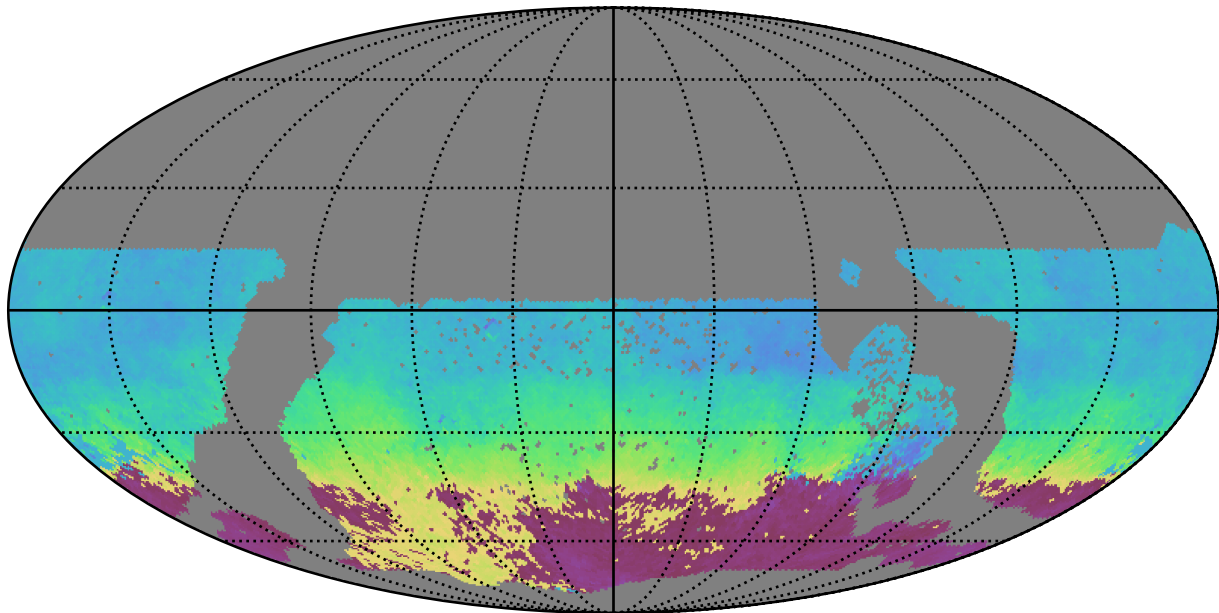
extra_ss_neo7_v3.4_10yrs WFD g band: AngleMean rotSkyPos
