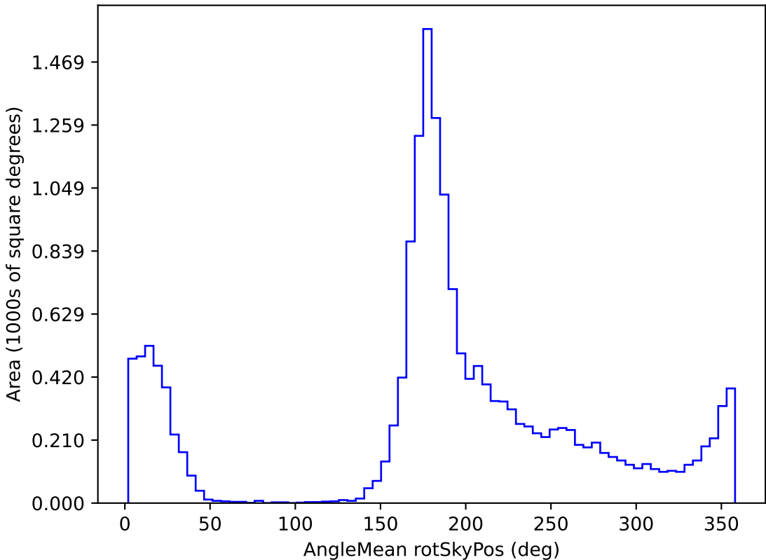
extra_ss_neo7_v3.4_10yrs WFD g band: AngleMean rotSkyPos
