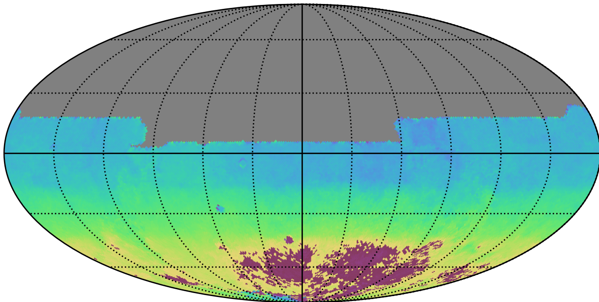
extra_ss_neo7_v3.4_10yrs All sky y band: AngleMean rotSkyPos
