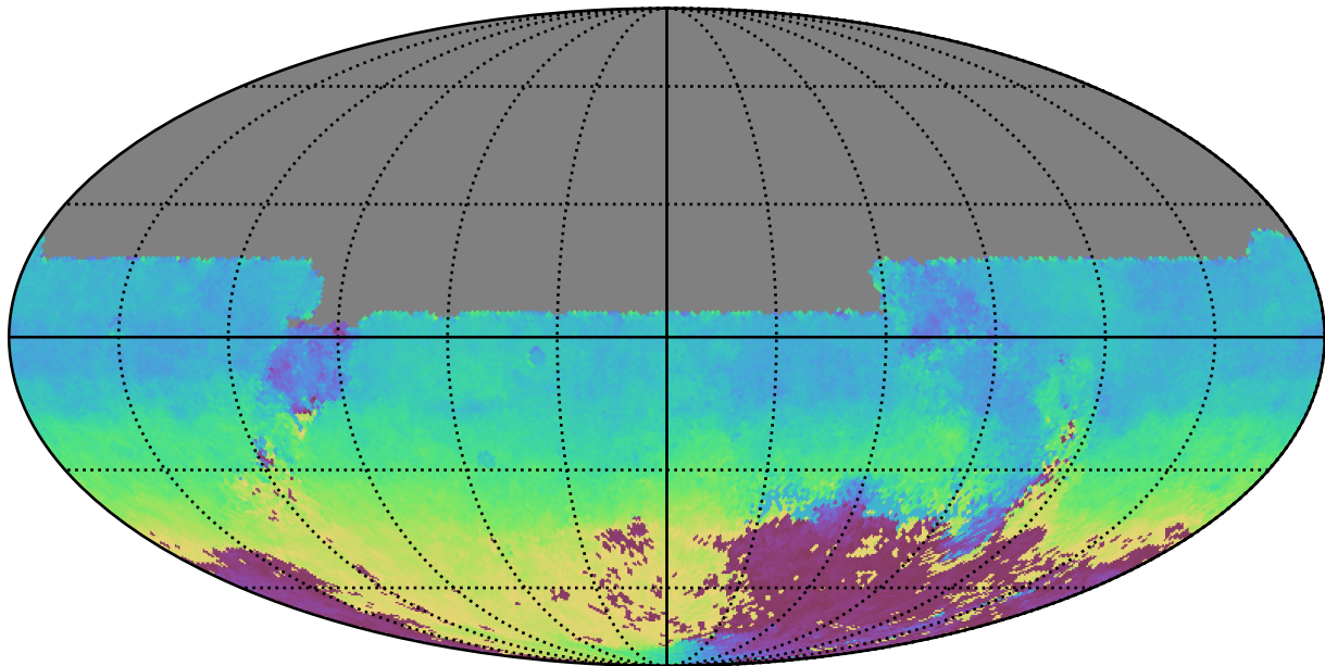
extra_ss_neo7_v3.4_10yrs All sky u band: AngleMean rotSkyPos
