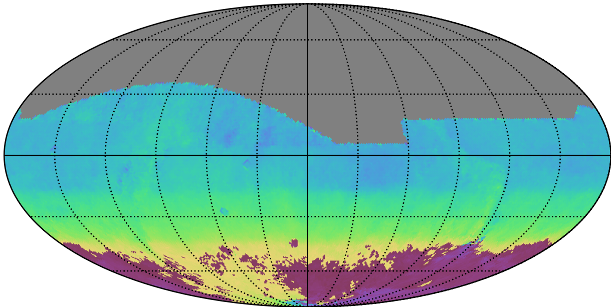
extra_ss_neo7_v3.4_10yrs All sky i band: AngleMean rotSkyPos
