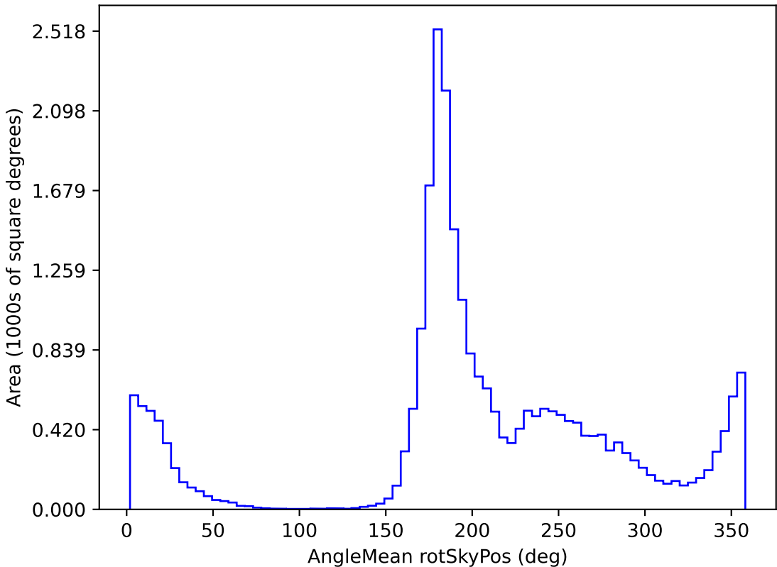
extra_ss_neo7_v3.4_10yrs All sky i band: AngleMean rotSkyPos
