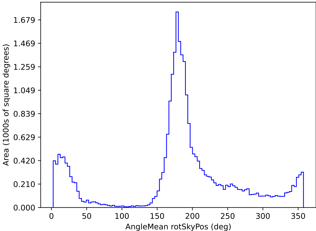
extra_ss_neo7_v3.4_10yrs All sky g band: AngleMean rotSkyPos
