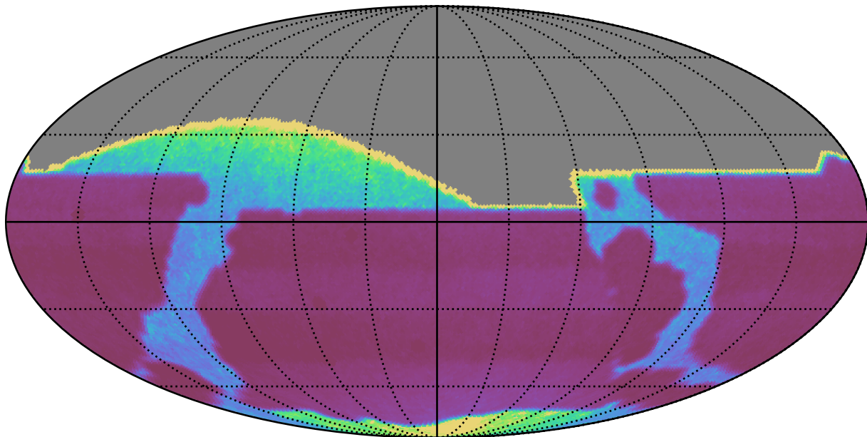
extra_ss_neo7_v3.4_10yrs : properMotion
