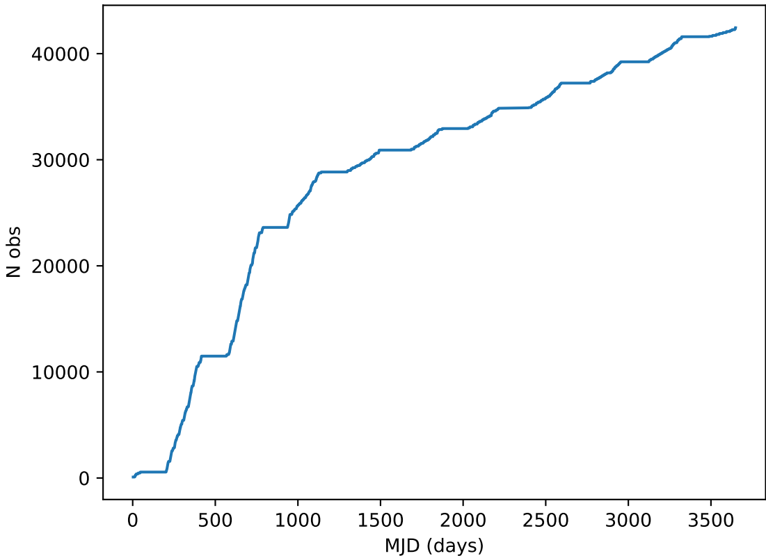
extra_ss_neo7_v3.4_10yrs note like DD:COSMOS%: Cumulative
