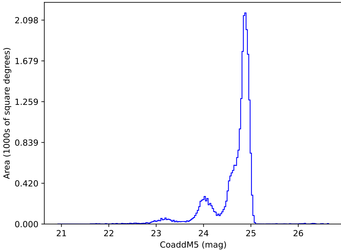
extra_ss_neo7_v3.4_10yrs y: CoaddM5
