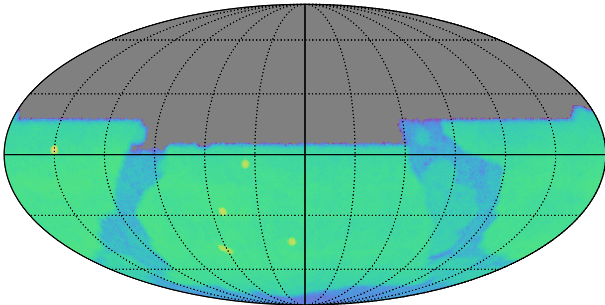
extra_ss_neo7_v3.4_10yrs u: CoaddM5
