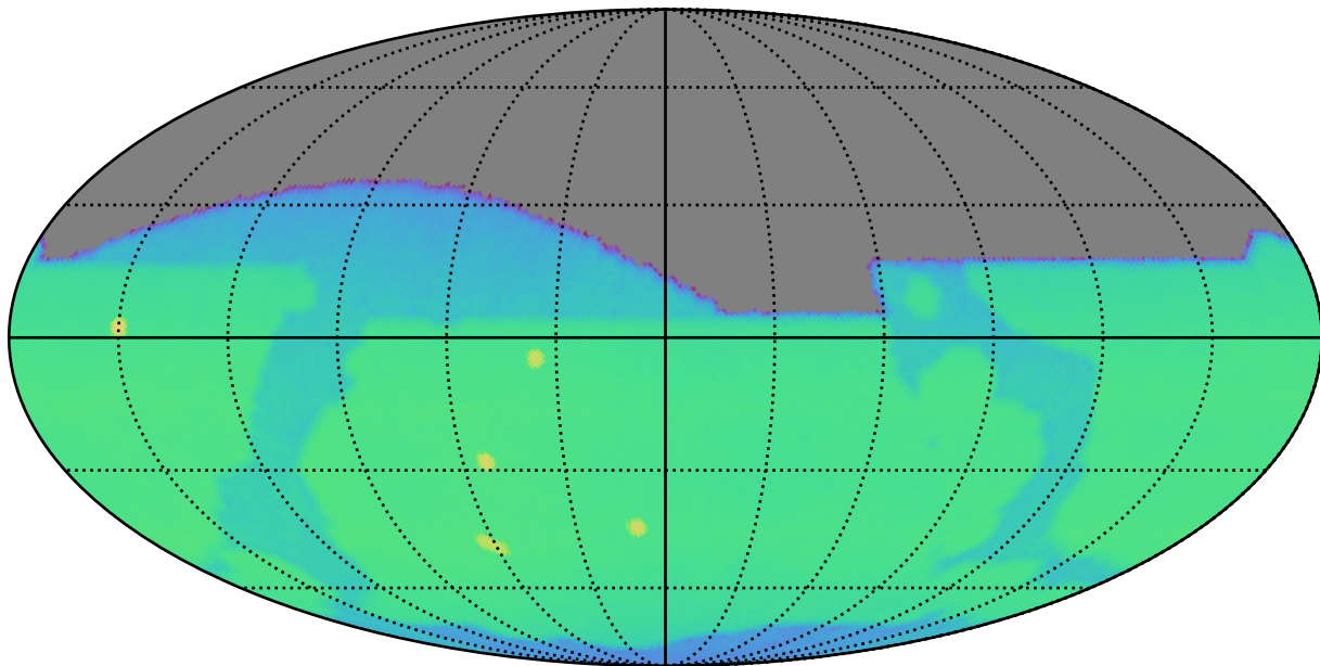
extra_ss_neo7_v3.4_10yrs i: CoaddM5
