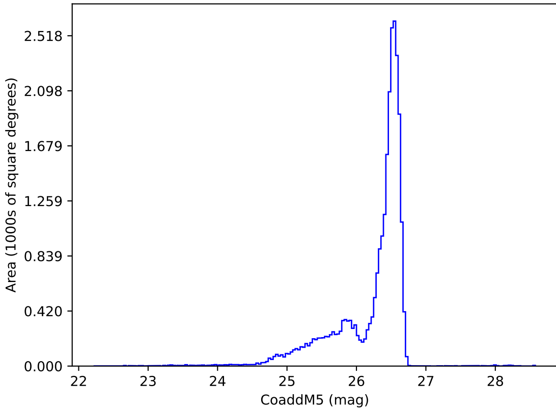
extra_ss_neo7_v3.4_10yrs i: CoaddM5
