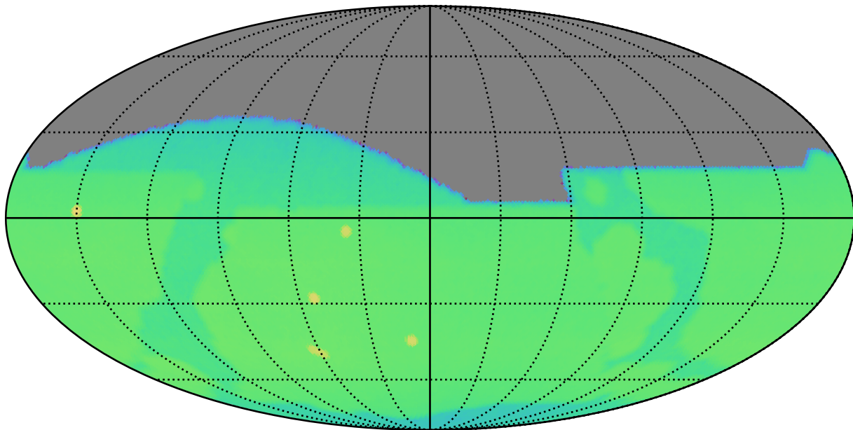
extra_ss_neo7_v3.4_10yrs : CoaddM5
