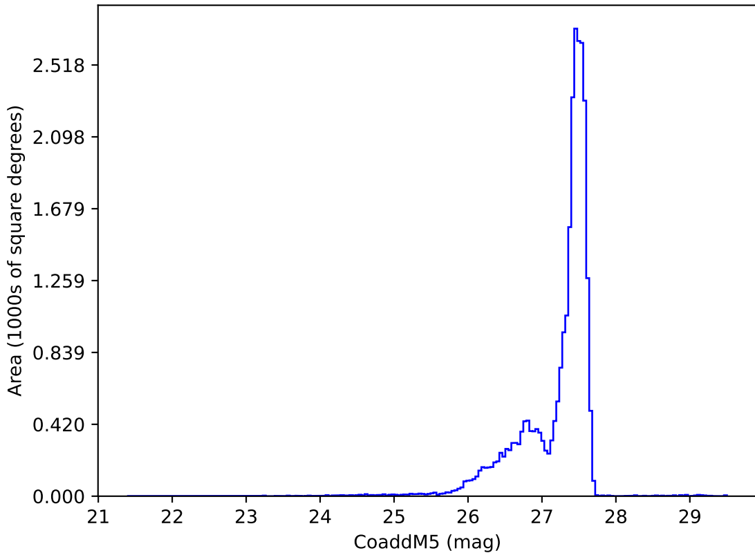
extra_ss_neo7_v3.4_10yrs : CoaddM5
