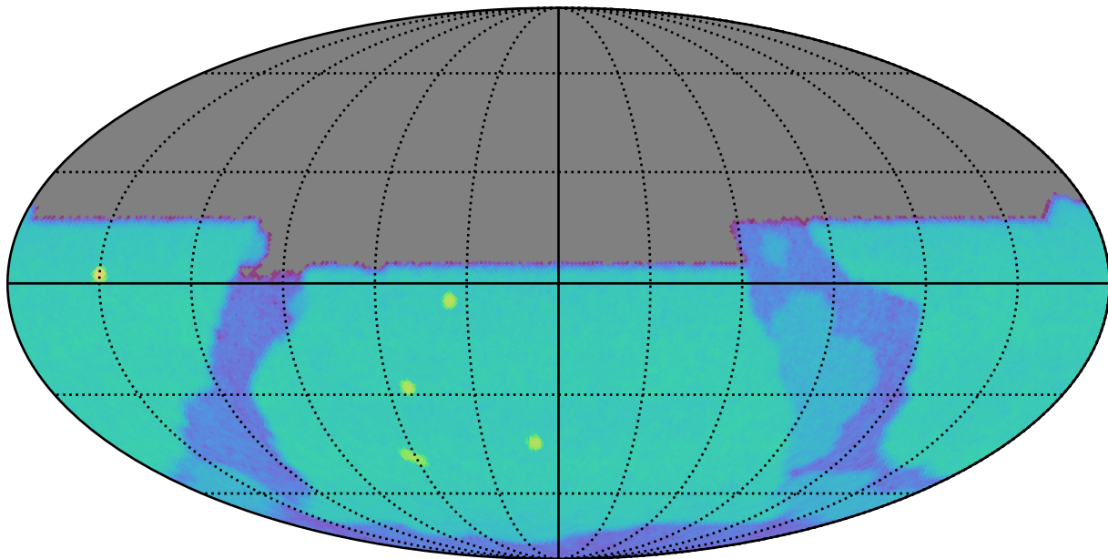
extra_ss_neo5_v3.4_10yrs u: SurfaceBrightLimit
