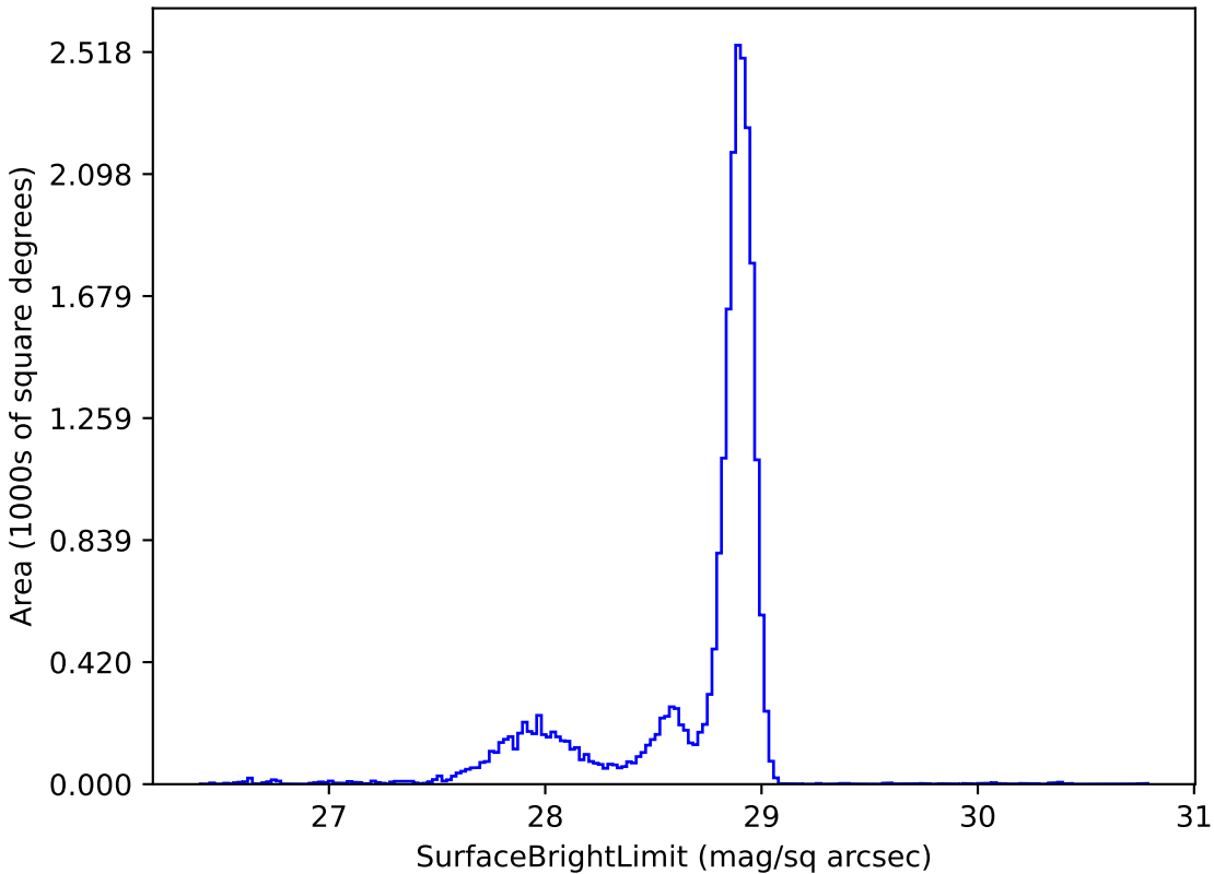
extra_ss_neo5_v3.4_10yrs u: SurfaceBrightLimit
