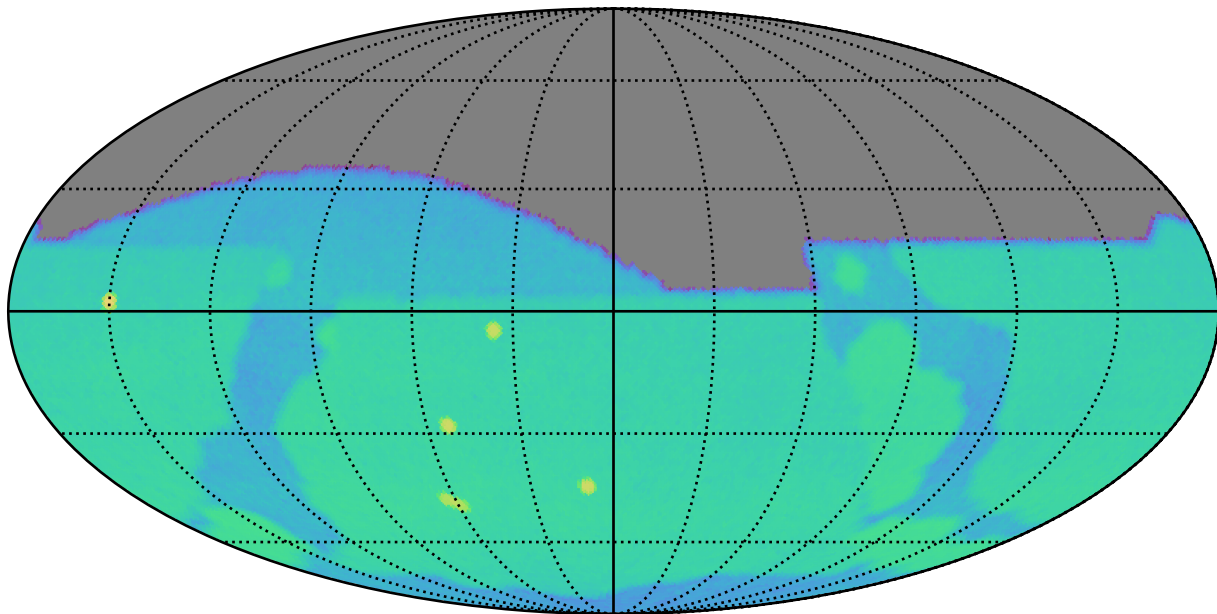
extra_ss_neo5_v3.4_10yrs g: SurfaceBrightLimit
