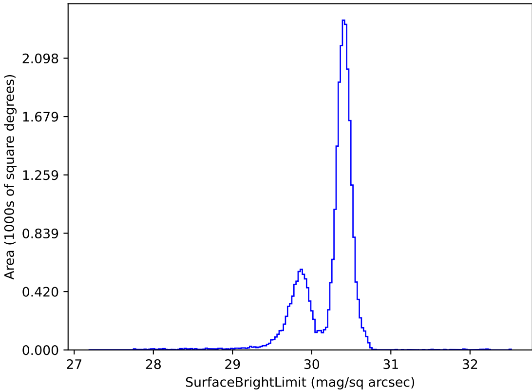
extra_ss_neo5_v3.4_10yrs g: SurfaceBrightLimit
