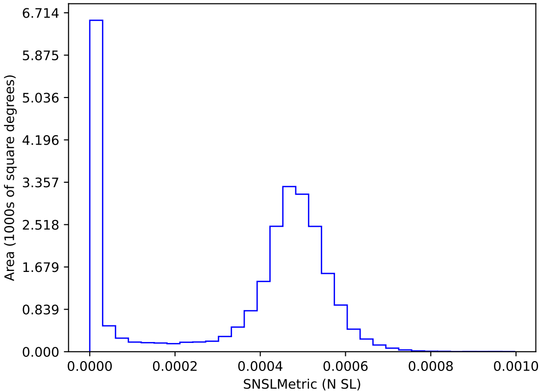
extra_ss_neo5_v3.4_10yrs : SNSLMetric
