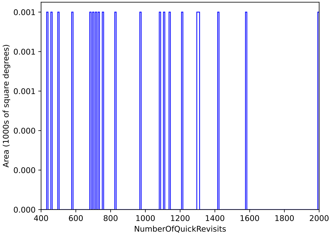
extra_ss_neo5_v3.4_10yrs : NumberOfQuickRevisits
