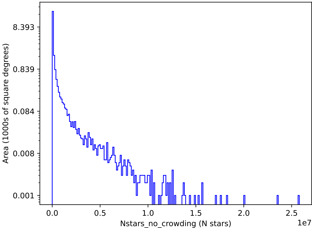
extra_ss_neo5_v3.4_10yrs y: Nstars_no_crowding
